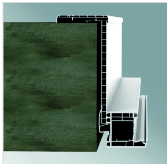
2 Laschensystem mit Kammerprofil an einer Fensterinnenlaibung
