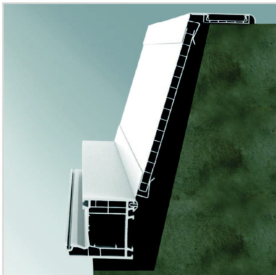
1 Variosystem mit Kammerprofil an einer Fensterinnenlaibung
